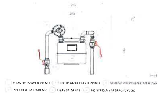
Detail meracej (domovej) regulačnej zostavy
